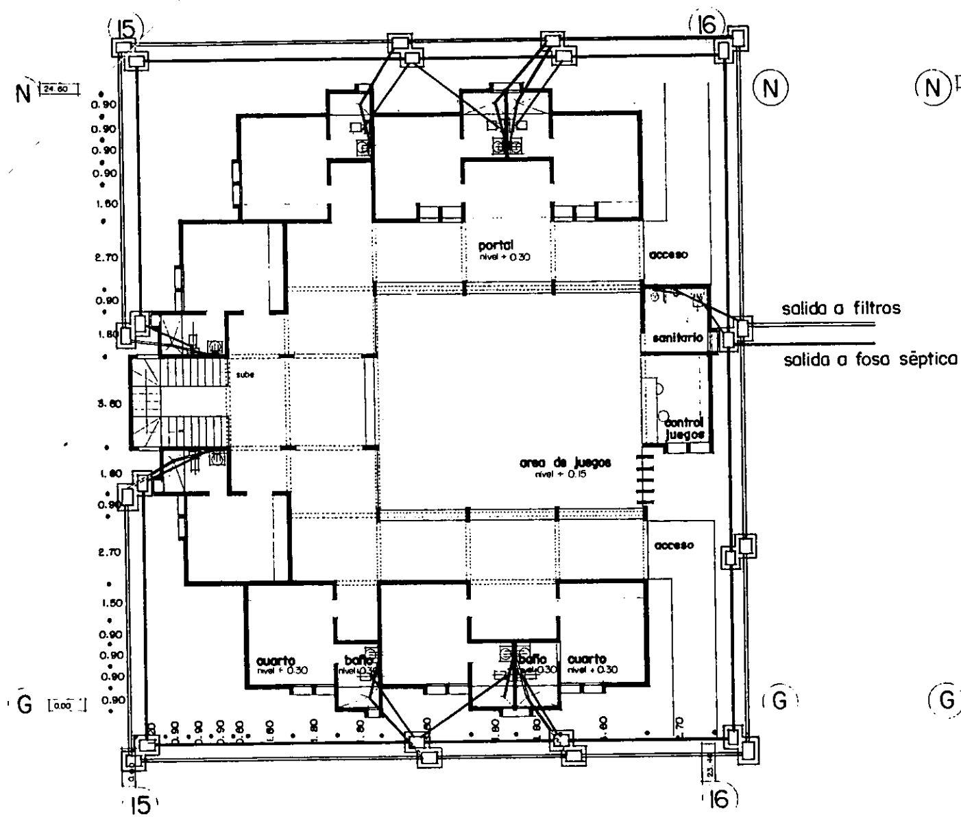
planta tipo de habitaciones
