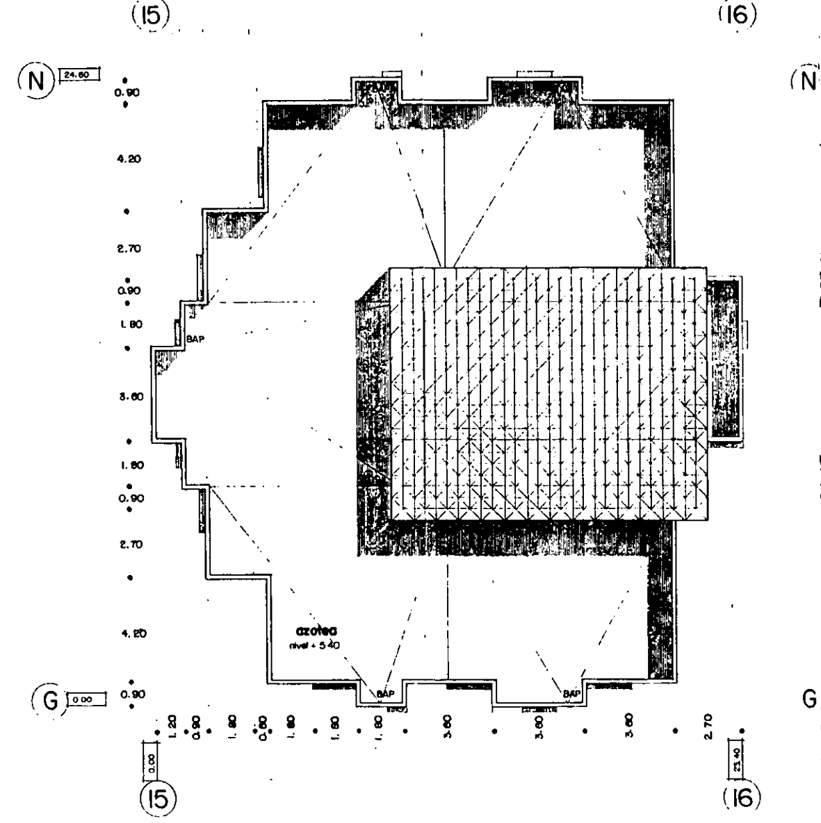
planta azotea
