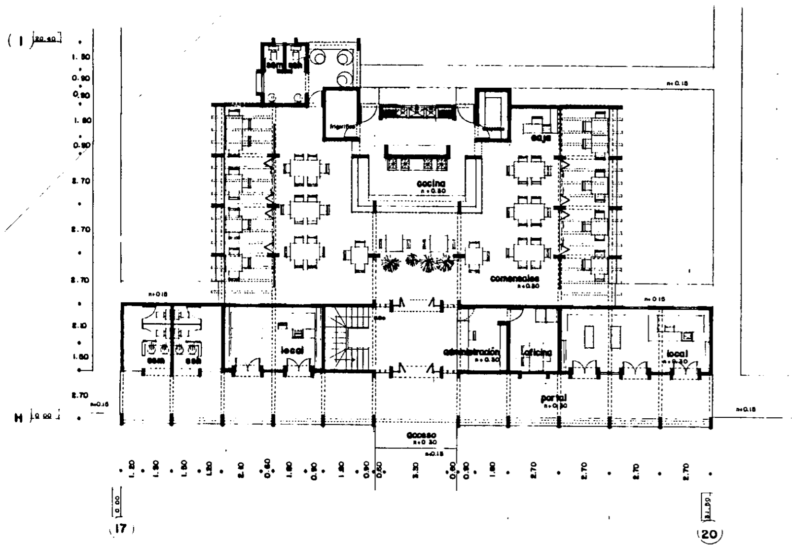
planta de restaurante y locales
