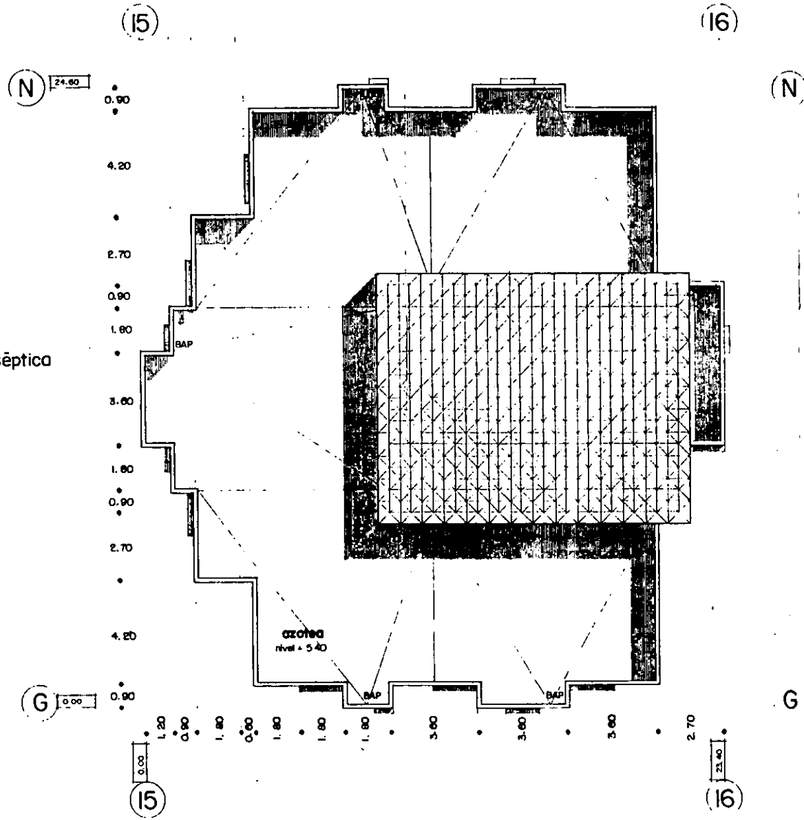
planta azotea
