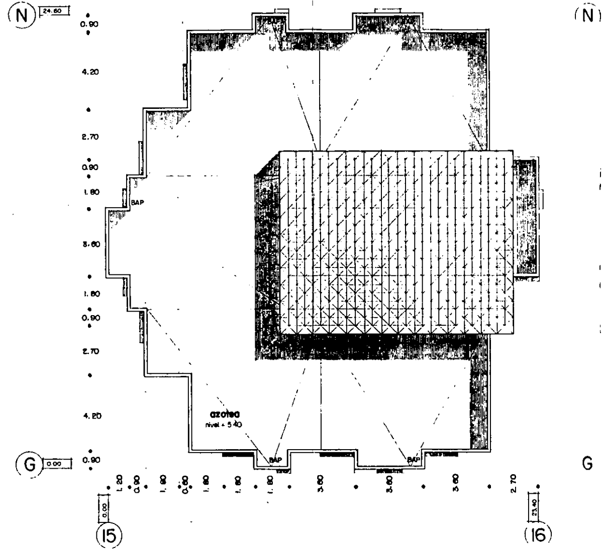
planta azotea
