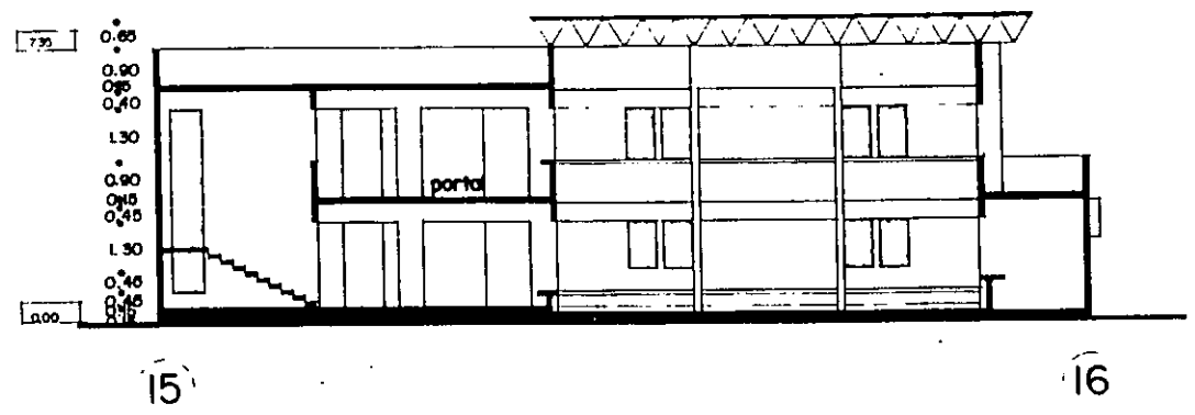
corte transversal
