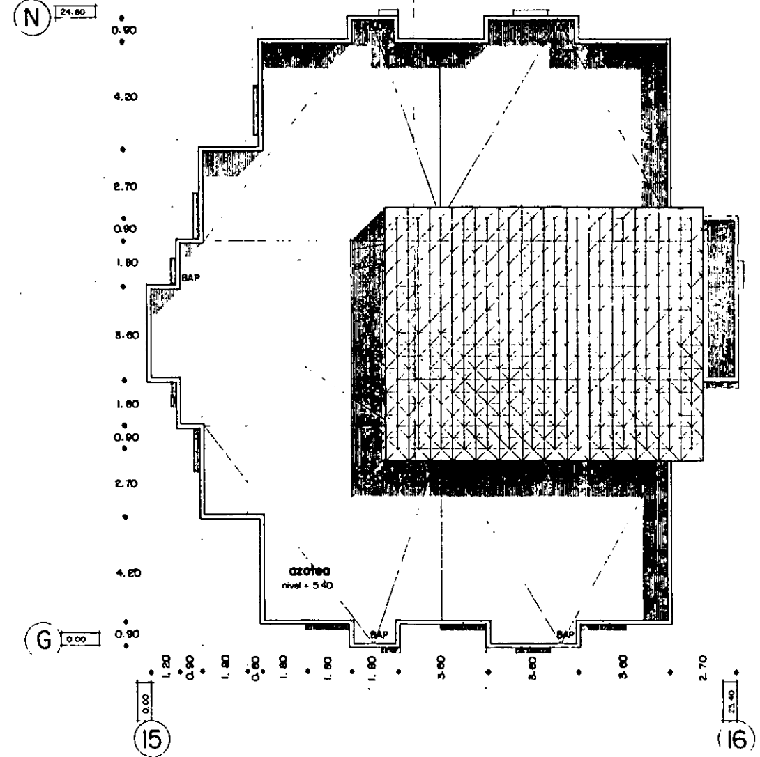
planta azotea
