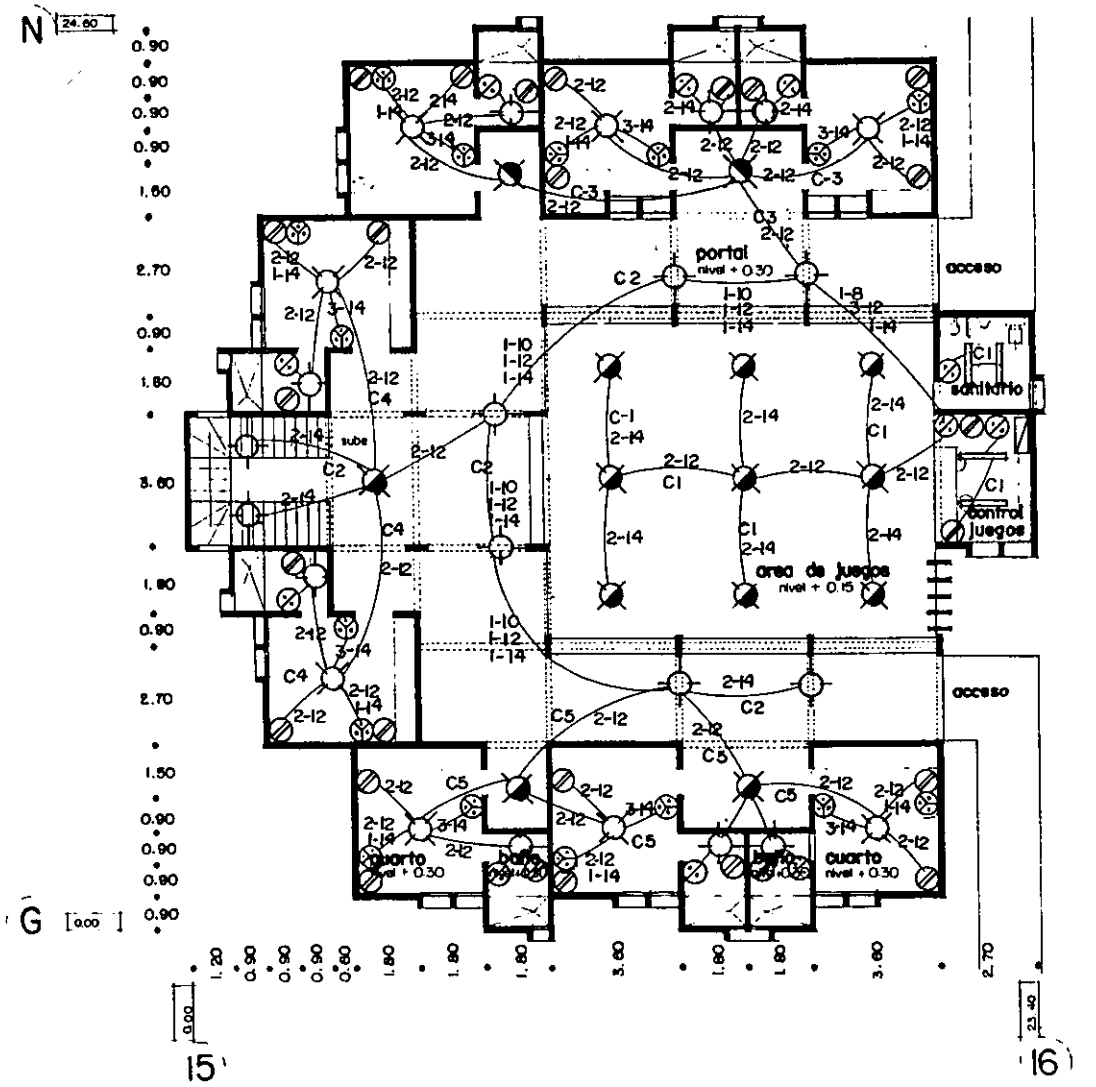
planta tipo de habitaciones
